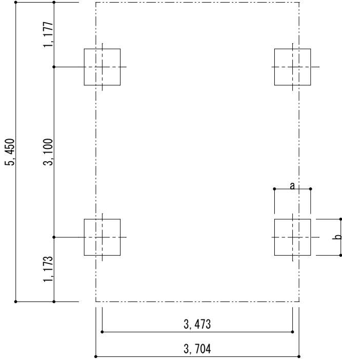
■ 基礎配置図
